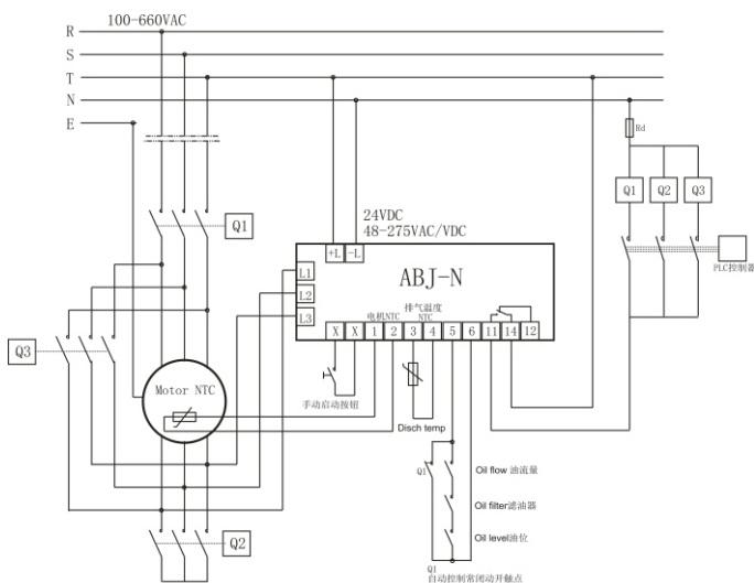
推荐电路2: Y~ \Delta 起动电路
