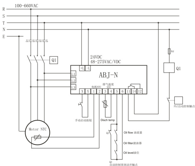
推荐电路1：直接起动
